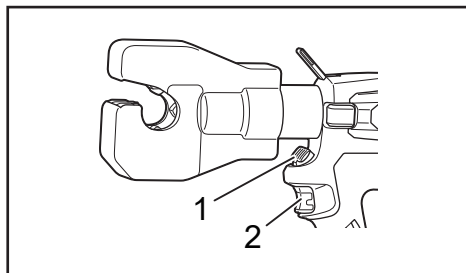
► 1. Vabastusnupp 2. Päästik
