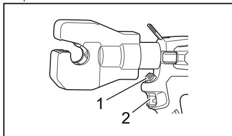
► 1. Frigørelsesknap 2. Afbryder
