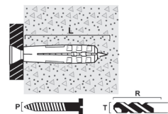
Lättbetong
