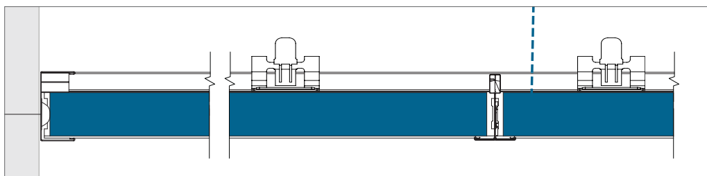
Väggavslutning med U-profil och väggfjäder.
