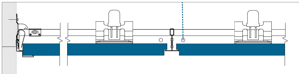
E-kant - kantavslutning med L-list och kantfjäder FIXT.
