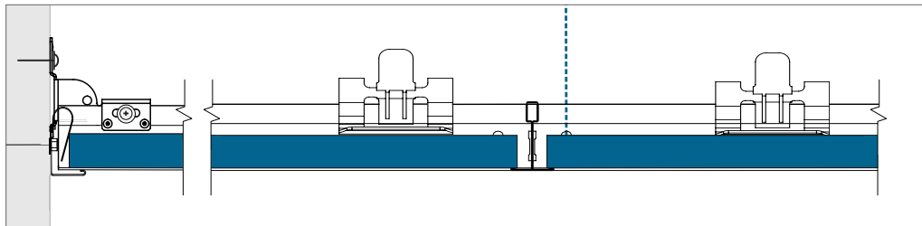
A-kant - kantavslutning med L-list och kantfjäder FIXT.
