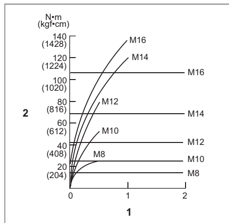
1. Kinnitamisaeg (sekund) 2. Väändemoment
