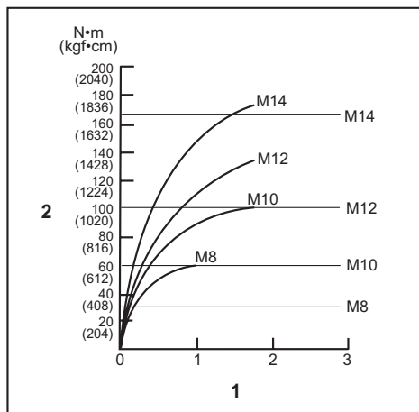
1. Pievilkšanas laiks (sekundēs) 2. Pievilkšanas griezes moments
